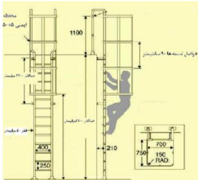
شکل ۱۷- نردبان ثابت با محفظه حفاظی
