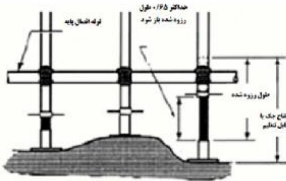
انکال ۵۱ - نحوه برپایی داربست
