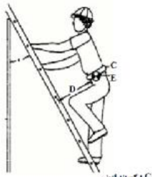
C: کمر بند ایمنی E: ابزار منوقف‌کننده سقوط D: فاصله جلوی فرد صعودکننده تا مرکز پایه نردبان
