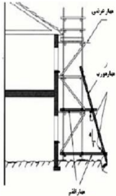
شکل ۴۲- مهار مورب داربست
